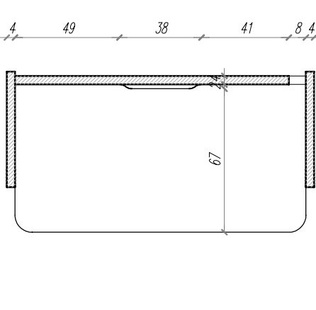
Przekrój na wysokości 65cm:
