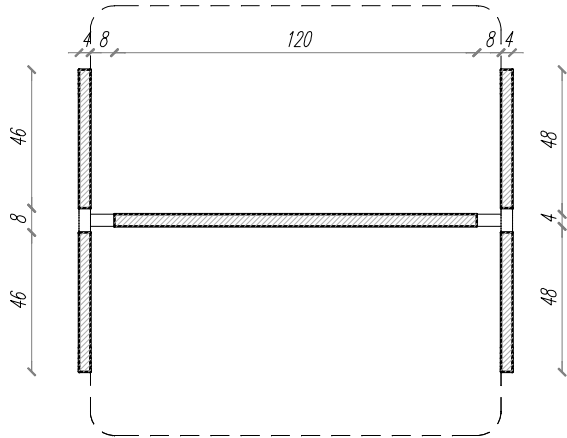
Przekrój na wysokości 65cm:
