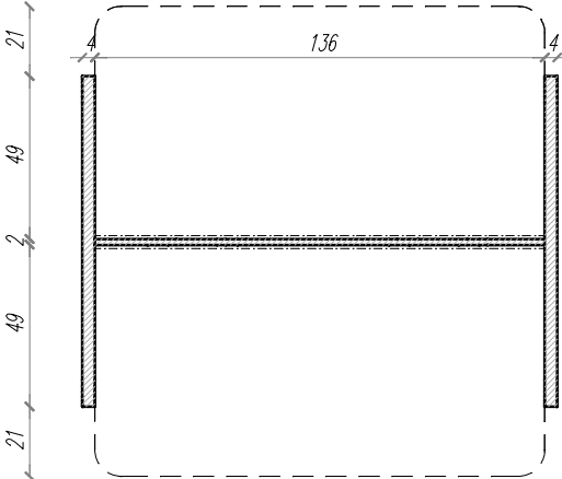
Przekrój na wysokości 15cm:
