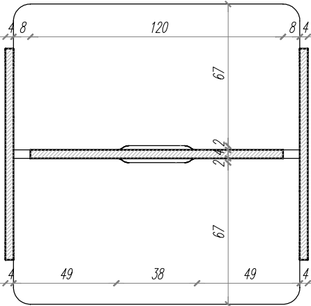
Przekrój na wysokości 80cm:
